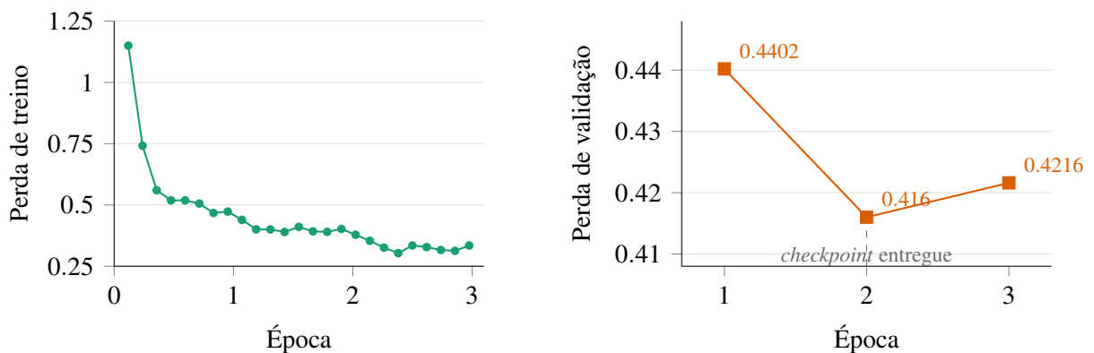
Figura 3 – Perdas de treino e de validação no ajuste supervisionado
