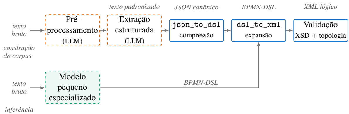
Figura 1 – Protocolo de compressão semântica: construção do corpus e inferência
