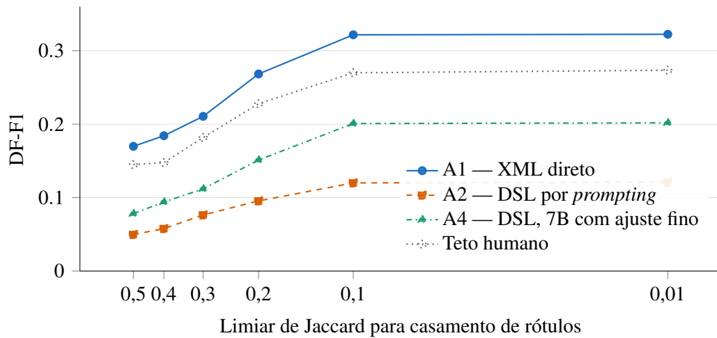
Figura 5 – Saturação do DF-F1 conforme o casamento de rótulos é afrouxado
