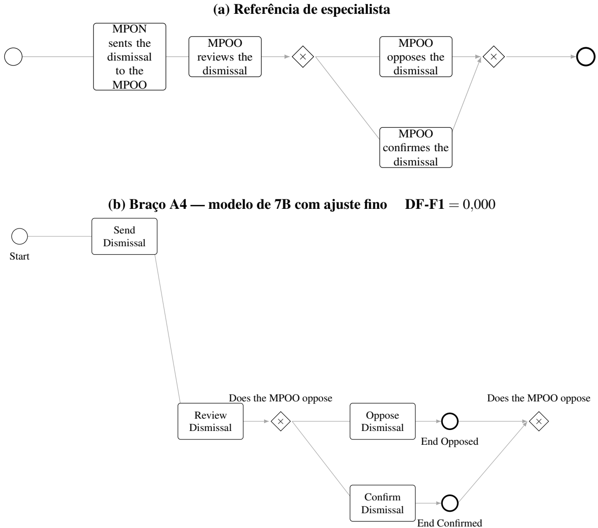
Figura 6 – Divergência de nomenclatura sem divergência de estrutura ( pmo_52 )
