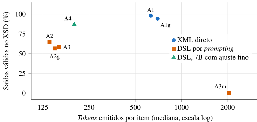
Figura 4 – Custo de saída contra validade sintática, por braço
