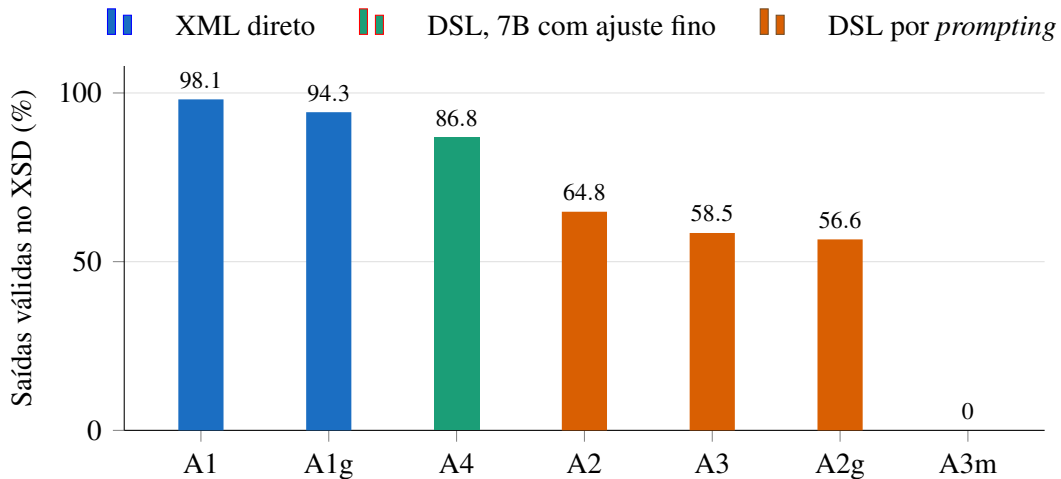
Figura 2 – Validade sintática por braço experimental
