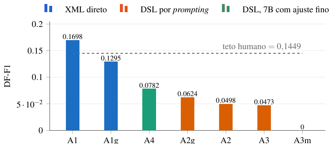
Figura 7 – Fidelidade topológica por braço, relativa à concordância entre especialistas
